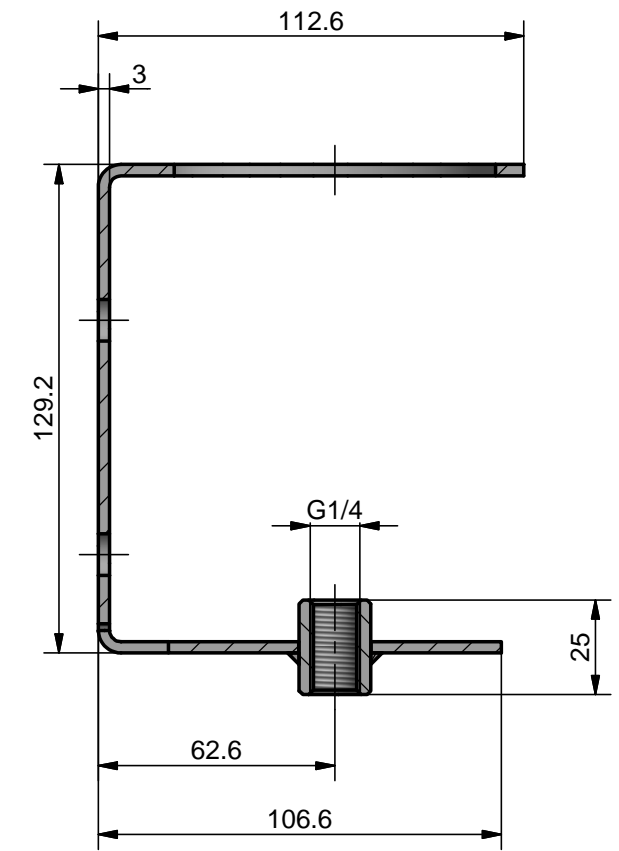
A-A ( 1 : 2 )
